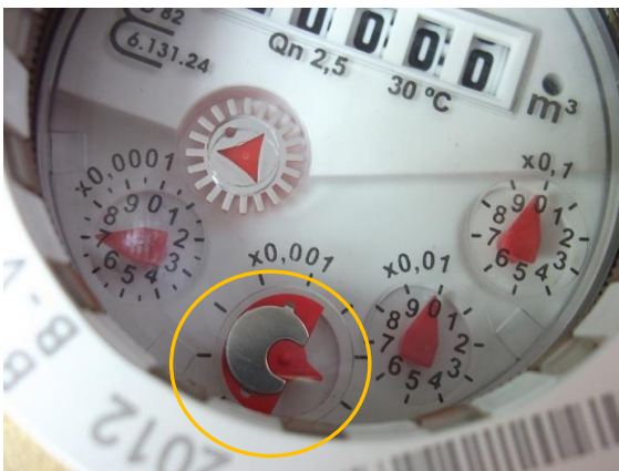
Reflektor-Zeiger im Nassbereich unter dem Glas
