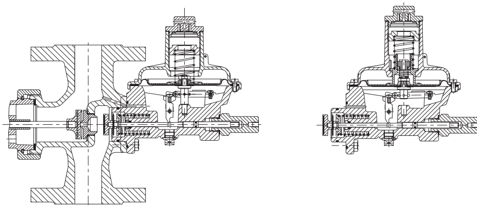
Abb. 2: Sicherheitsabsperrentil Typ I - pdsu
