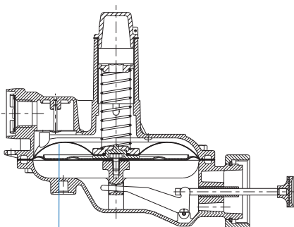
integrierte Sicherheitsmembrane
