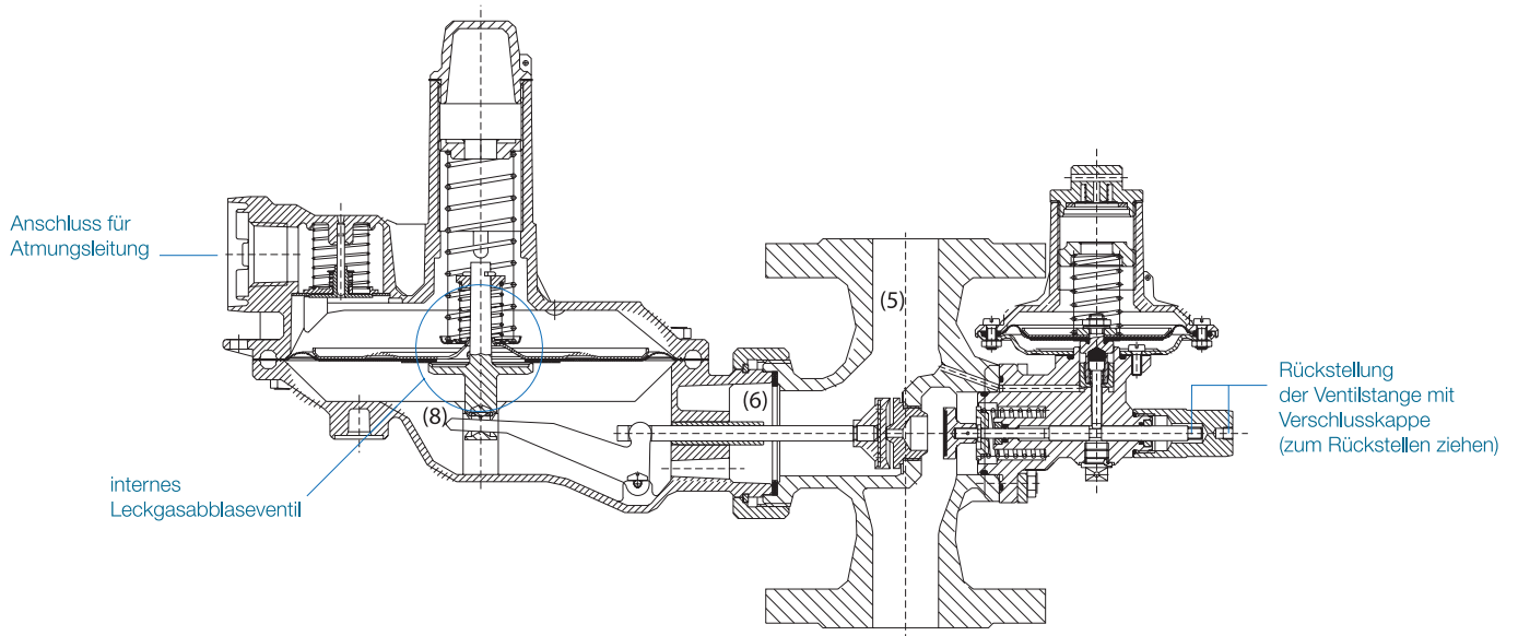
Abb.1: Gasdruckregelgerät 133 mit integriertem Leckgas-Abblaseventil und Sicherheitsabsperrentil Typ 033 pdsu
