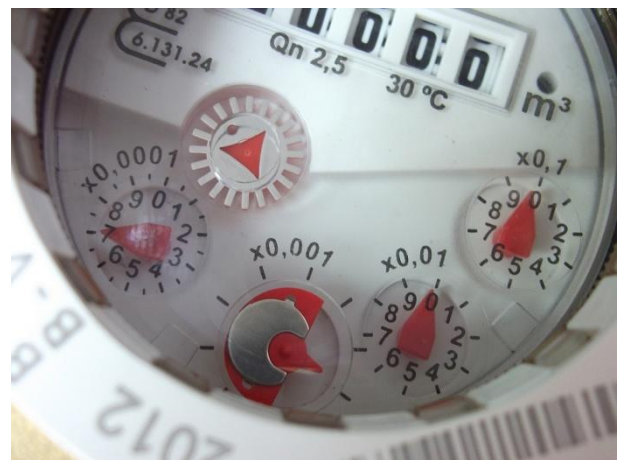
Reflektor-Zeiger im Nassbereich unter dem Glas
