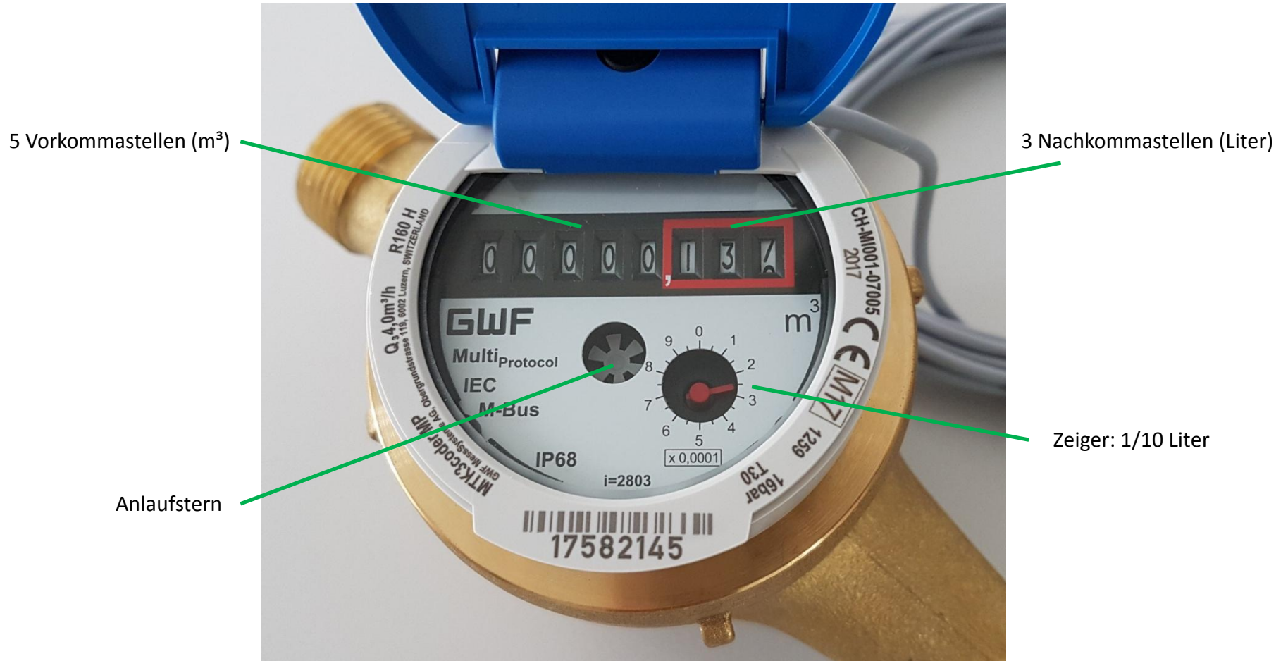
Mehrstrahl-Trockenläufer mit Absolut-Encoder IP68
