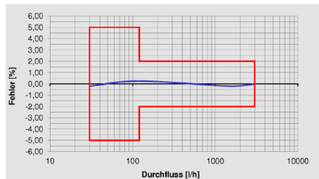
Typische Fehlerkurve für Qn1,5 Klasse B
