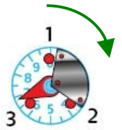
Target abseits
