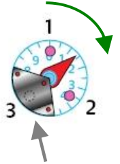
Target präsent
